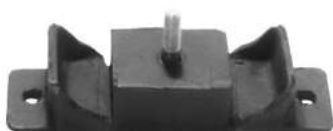
Código: 80114 Modelo: R. 4 - R. 6 Nº Original: 1016092 Soporte delantero derecho e izquierdo
